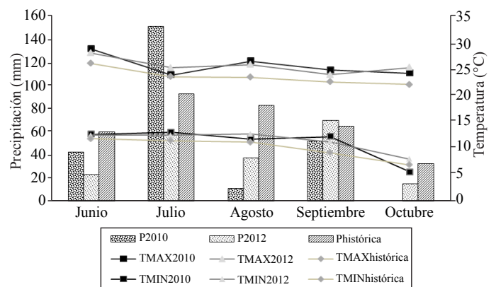
Figura 1. Precipitación mensual (mm) y temperaturas (°C) máximas y mínimas) en el Campo Experimental Zacatecas en los años 2010 y 2012.
