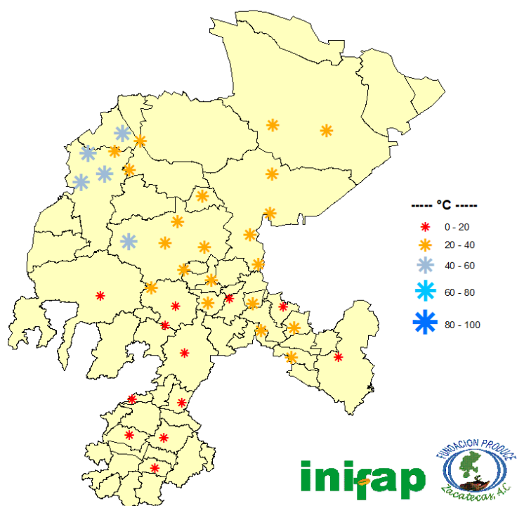
Figura 3. Horas frío acumuladas en la segunda decena del mes de noviembre del 2019.
