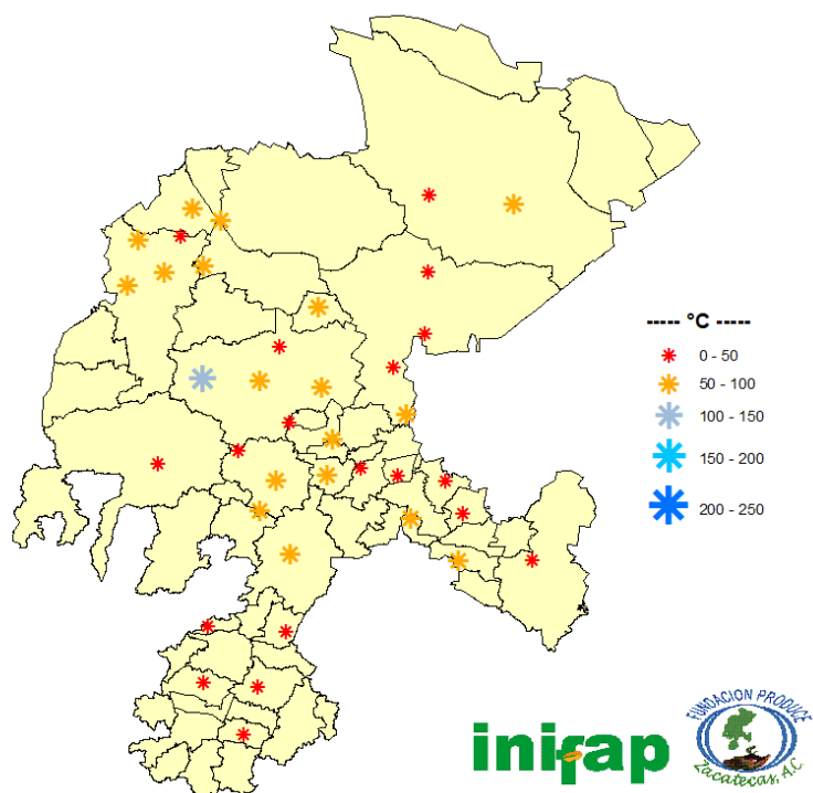
Figura 5. Horas frío acumuladas en el mes de noviembre del 2019.
