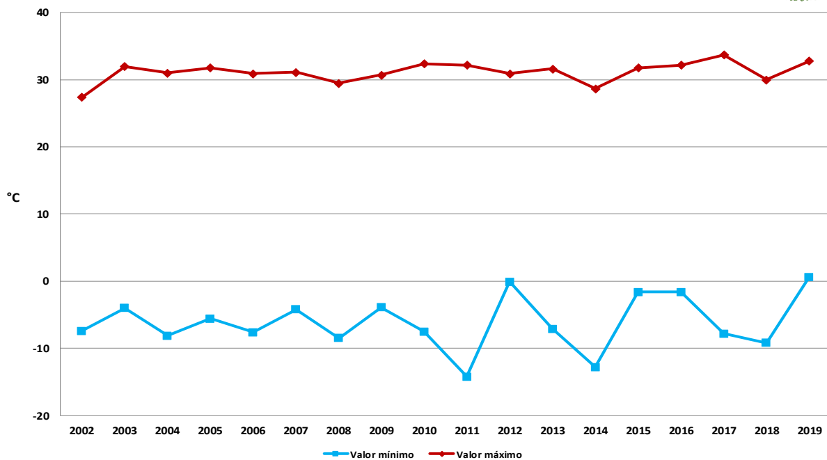
Figura 9. Valores máximos y mínimos históricos de temperatura en el mes de noviembre, considerando las 38 estaciones de la Red de monitoreo agroclimático del estado de Zacatecas.
