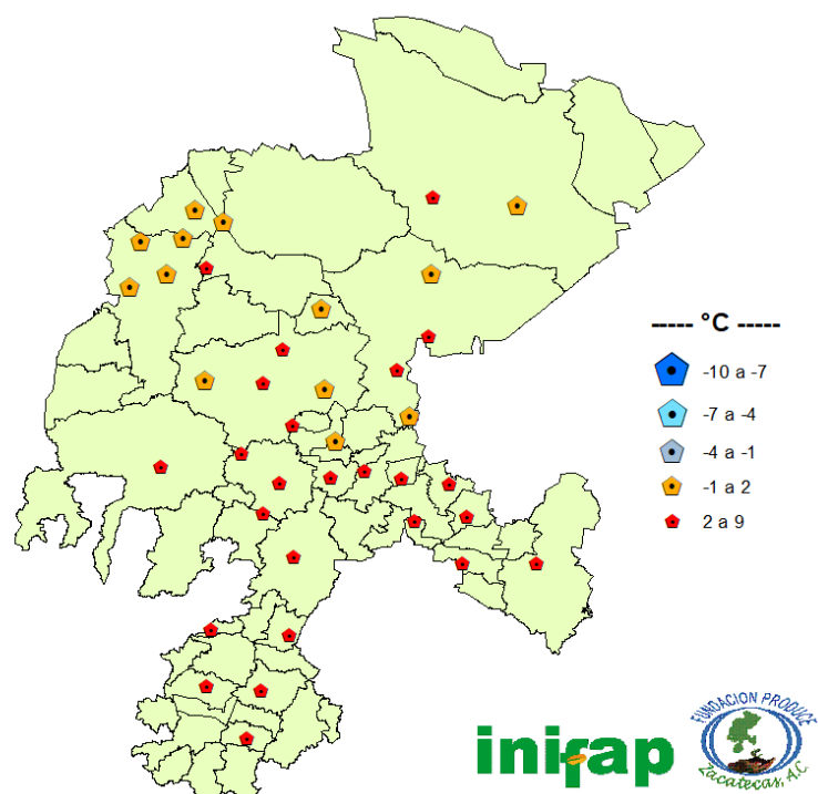
Figura 7. Valores mínimos de temperatura registrados en el mes de noviembre del 2019.
