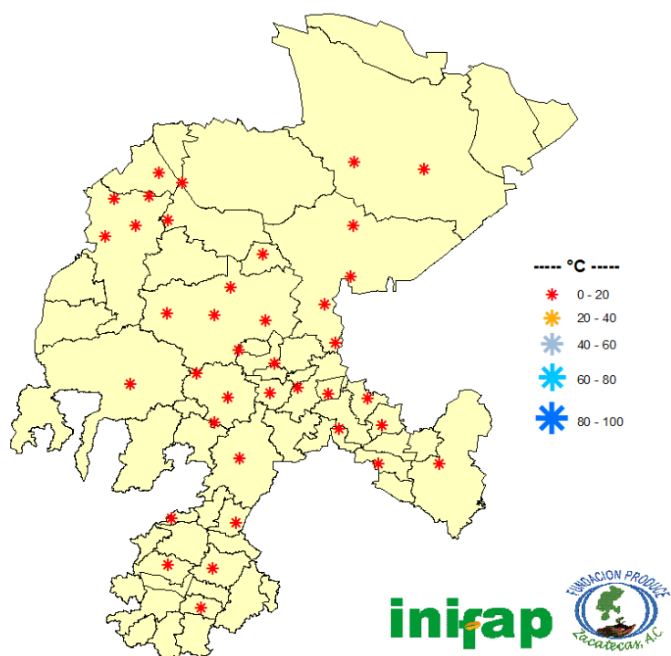
Figura 2. Horas frío acumuladas en la primera decena del mes de noviembre del 2019.
