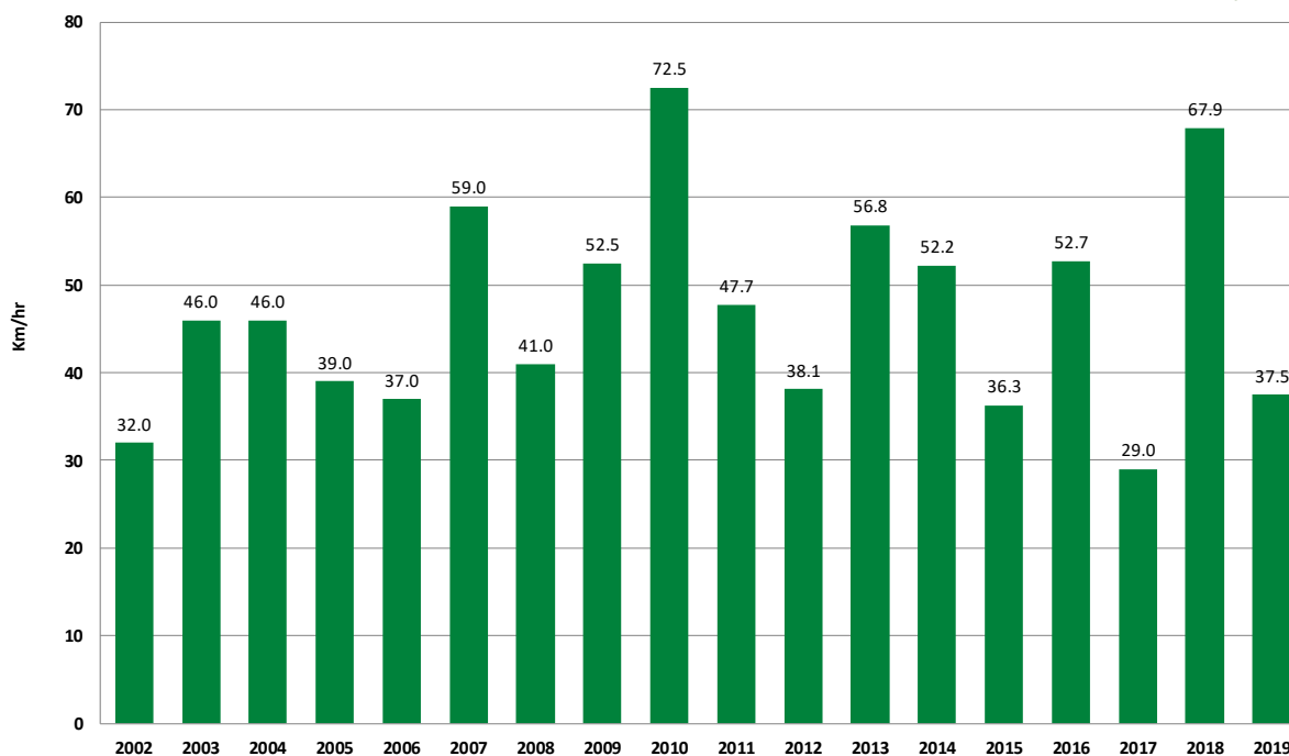
Figura 10. Valor máximo histórico de velocidad del viento en el mes de noviembre, considerando las 38 estaciones de la Red de monitoreo agroclimático del estado de Zacatecas.
