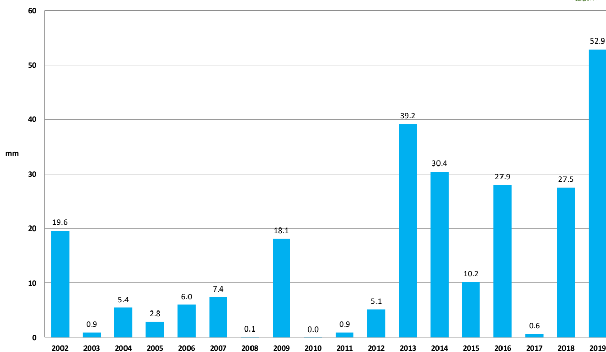
Figura 11. Precipitación promedio histórica del mes de noviembre considerando las 38 estaciones de la Red de monitoreo agroclimático del estado de Zacatecas.
