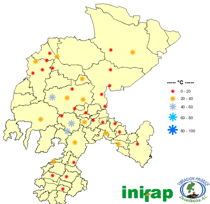
Figura 4. Horas frío acumuladas en la tercera decena del mes de noviembre del 2019.
