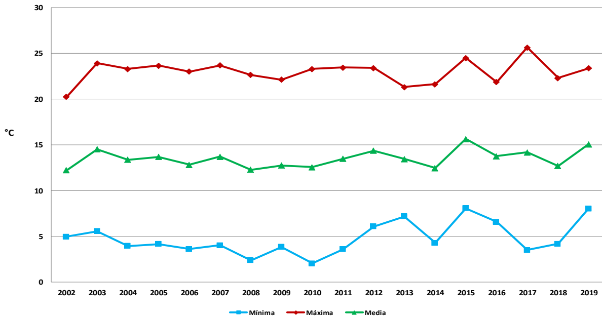
Figura 8. Temperatura media histórica en el mes de noviembre, considerando las 38 estaciones de la Red de monitoreo agroclimático del estado de Zacatecas.
