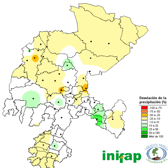
Figura 15. Desviación de la precipitación (%) ocurrida en los meses de junio a agosto de 2018 con respecto al promedio histórico.
