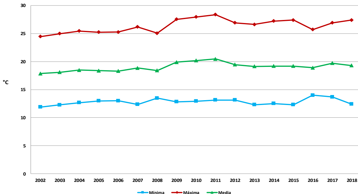
Figura 18. Temperatura promedio histórica en el mes de agosto, considerando las 38 estaciones de la red de monitoreo agroclimático del estado de Zacatecas.
