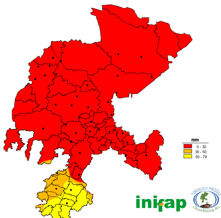
Figura 6. Precipitación de la primera decena del mes de agosto de 2018. Red de monitoreo agroclimático del estado de Zacatecas.
