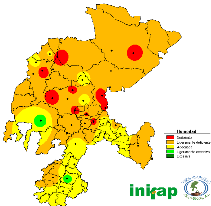
Figura 17. Índice de humedad del mes de agosto del 2018.
