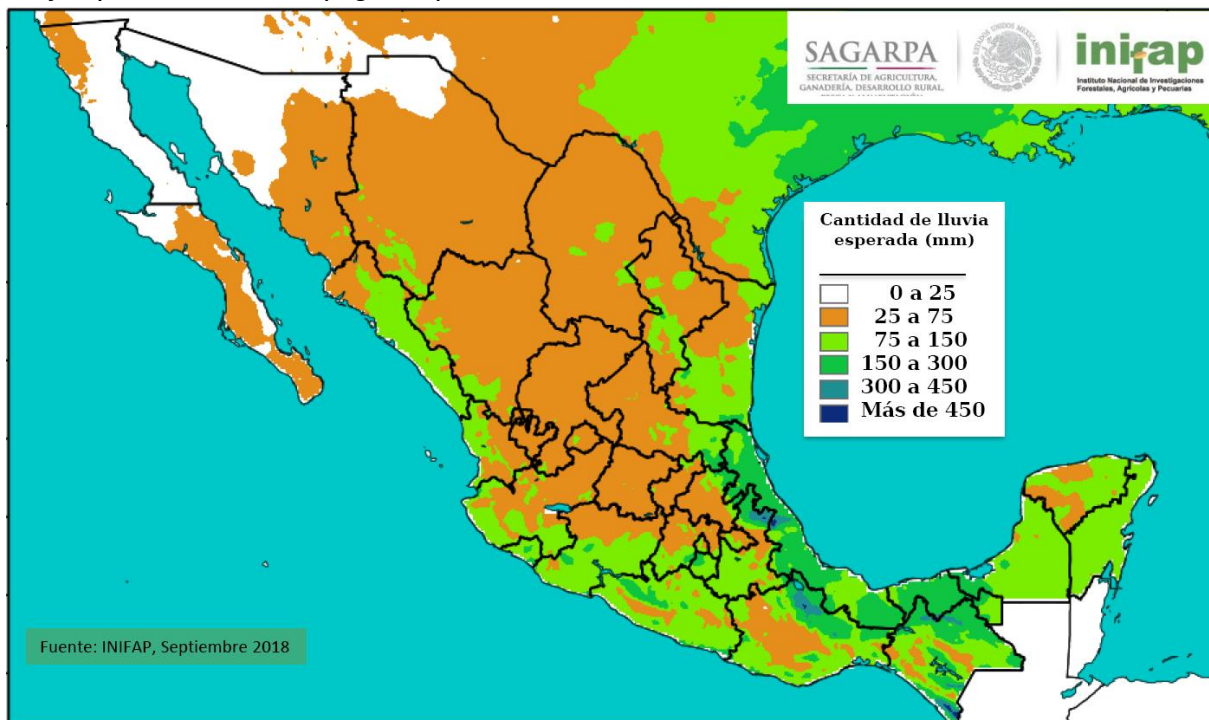
Figura 4. Pronóstico de lluvia para el mes de octubre de 2018.
