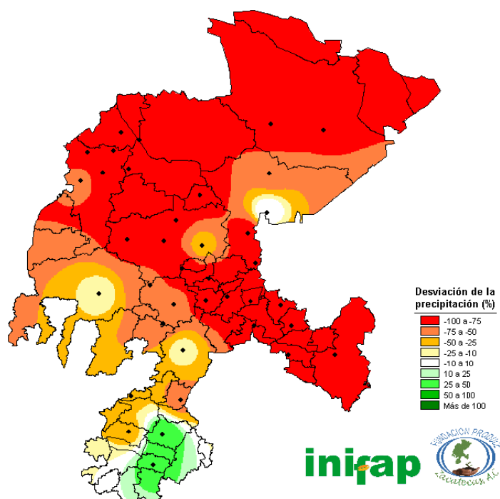
Figura 7. Desviación de la precipitación (%) ocurrida en la primera decena en agosto de 2018 con respecto al promedio histórico. Red de monitoreo agroclimático del estado de Zacatecas.
