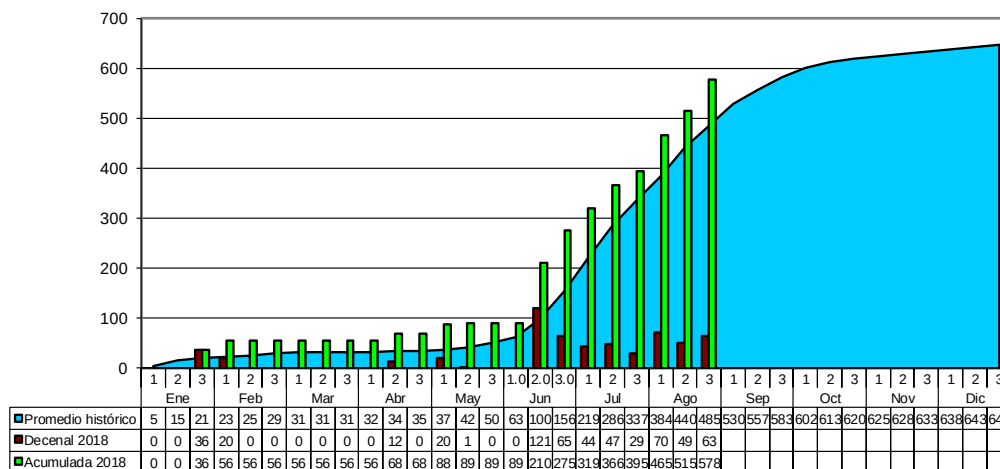
Figura 16. Precipitación decenal (arriba) y acumulada (abajo) hasta el mes de agosto en la estación UPSZ El Remolino, Juchipila. Red de monitoreo agroclimático del estado de Zacatecas.
