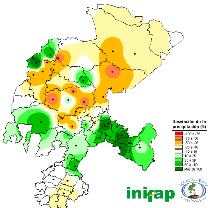
Figura 9. Desviación de la precipitación (%) ocurrida en la segunda decena de agosto de 2018 con respecto al promedio histórico. Red de monitoreo agroclimático del estado de Zacatecas.
