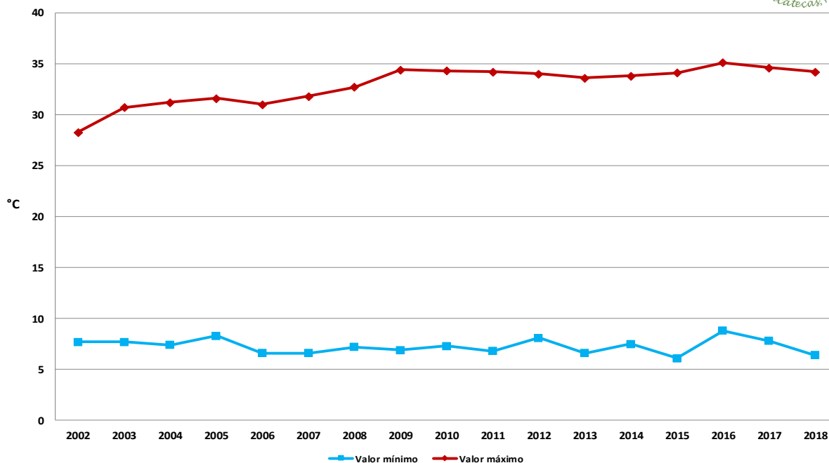
Figura 19. Valores máximos y mínimos históricos de temperatura en el mes de agosto, considerando las 38 estaciones de la red de monitoreo agroclimático del estado de Zacatecas.
