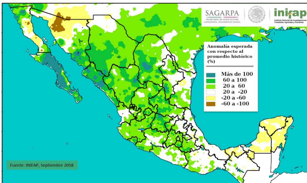
Figura 5. Pronóstico de anomalía de lluvia para el mes de octubre de 2018.
