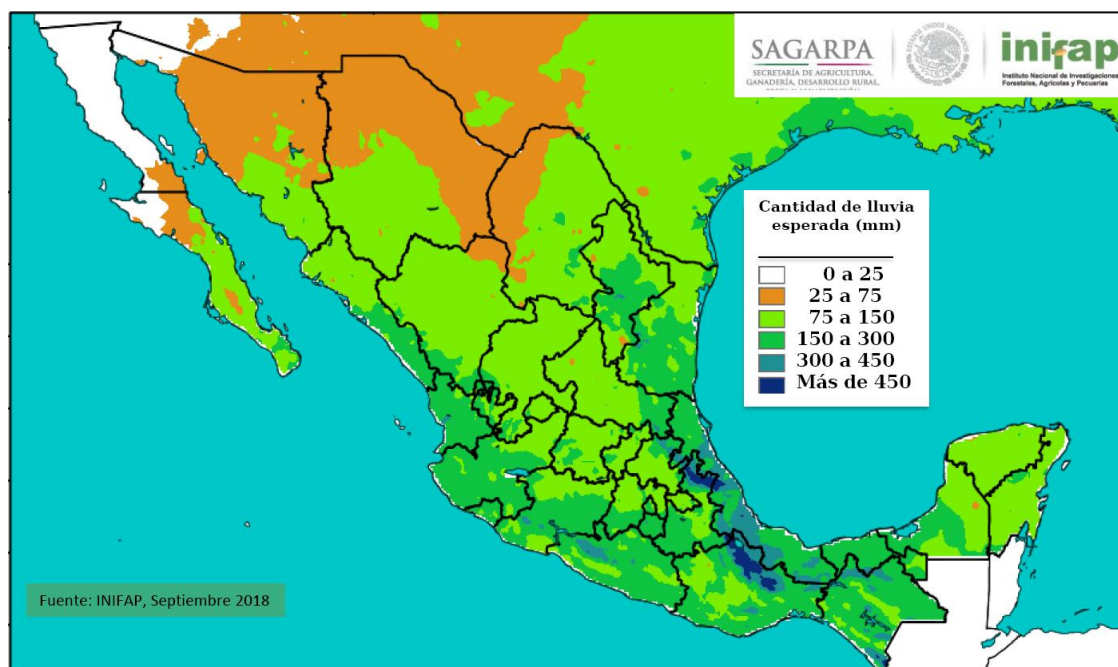
Figura 2. Pronóstico de lluvia para el mes de septiembre de 2018.
