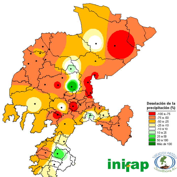
Figura 11. Desviación de la precipitación (%) ocurrida en la tercera decena de agosto de 2018 con respecto al promedio histórico. Red de monitoreo agroclimático del estado de Zacatecas.
