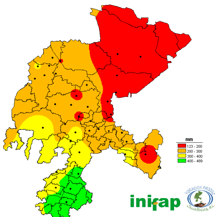
Figura 14. Precipitación acumulada en los meses de junio a agosto de 2018.
