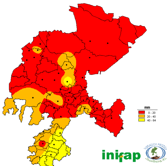
Figura 10. Precipitación de la tercera decena del mes de agosto de 2018. Red de monitoreo agroclimático del estado de Zacatecas.
