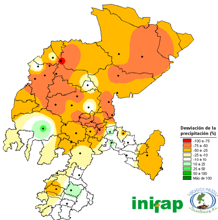
Figura 13. Desviación de la precipitación (%) ocurrida en el mes de agosto de 2018 con respecto al promedio histórico. Red de monitoreo agroclimático del estado de Zacatecas.
