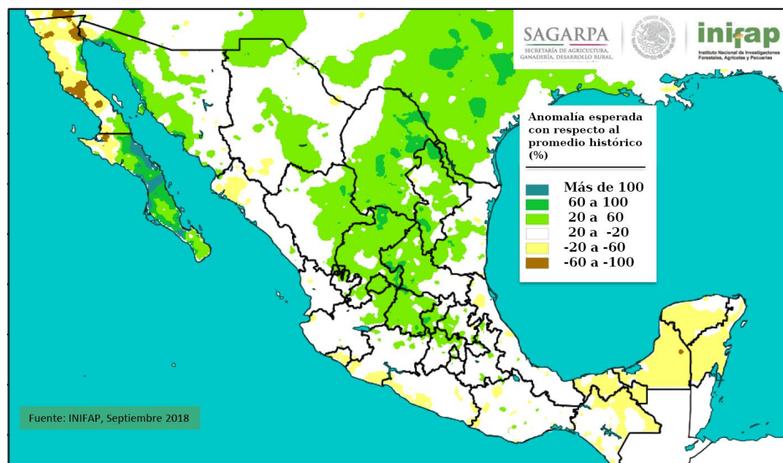
Figura 3. Pronóstico de anomalía de lluvia para el mes de septiembre de 2018.
