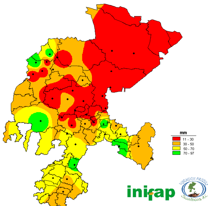
Figura 8. Precipitación de la segunda decena del mes de agosto de 2018. Red de monitoreo agroclimático del estado de Zacatecas.
