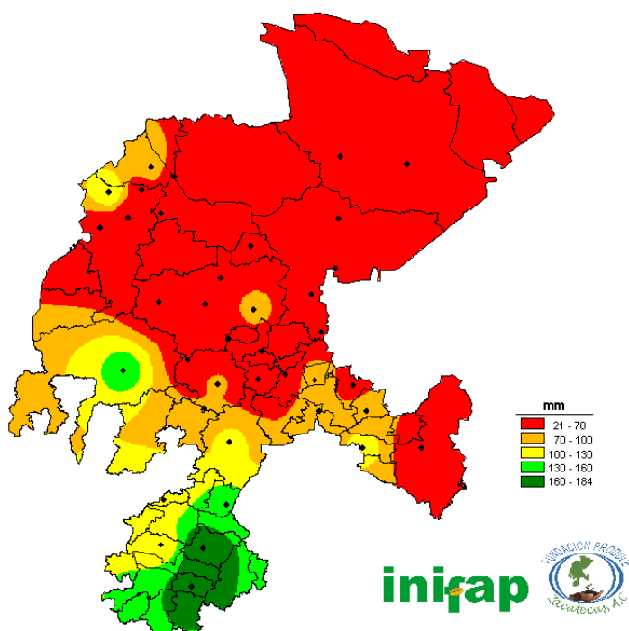
Figura 12. Precipitación del mes de agosto de 2018. Red de monitoreo agroclimático del estado de Zacatecas.
