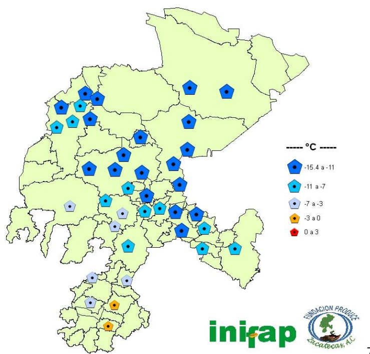
Figura 8. Valores mínimos de temperatura registrados en el mes de enero del 2018.
