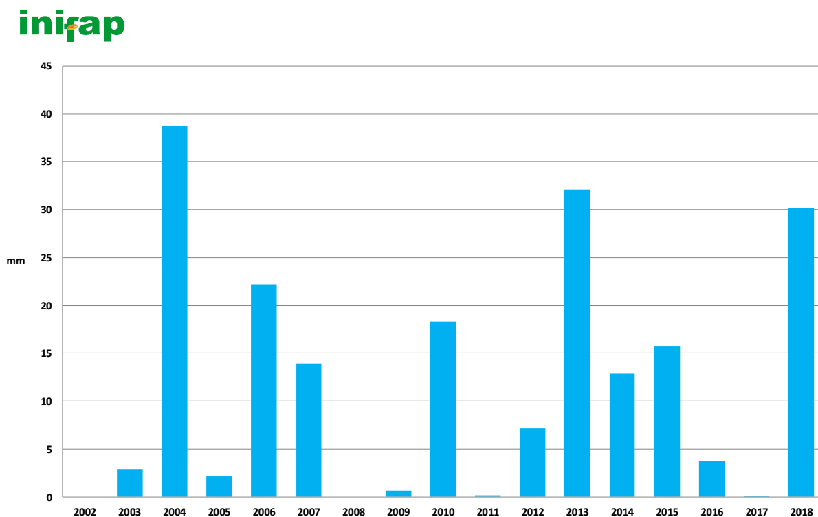
Figura 12. Precipitación promedio histórica del mes de enero considerando las 38 estaciones de la red de monitoreo agroclimático del estado de Zacatecas.
