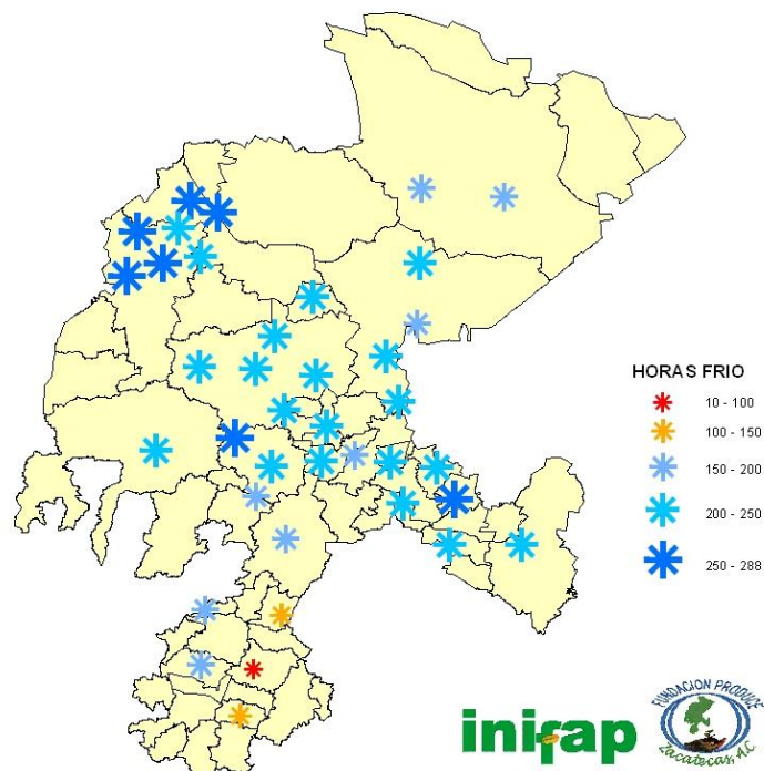
Figura 5. Horas frío acumuladas en el mes de enero del 2018.
