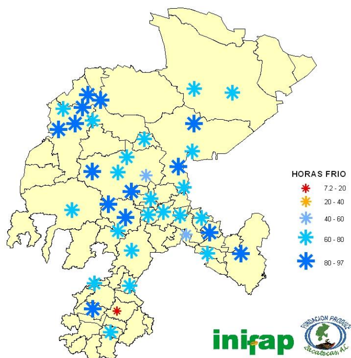
Figura 3. Horas frío acumuladas en la segunda decena del mes de enero del 2018.
