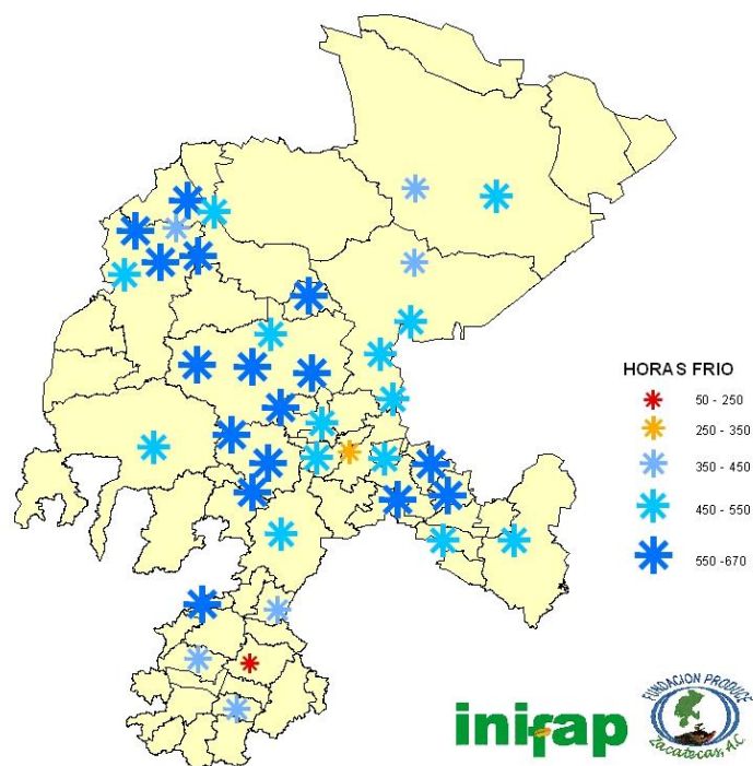
Figura 6. Horas frío acumuladas en los meses de noviembre 2017 a enero de 2018.
