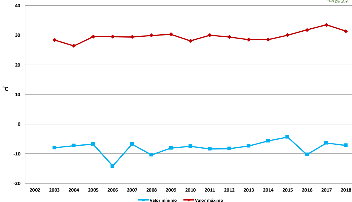
Figura 10. Valores máximos y mínimos históricos de temperatura en el mes de enero, considerando las 38 estaciones de la red de monitoreo agroclimático del estado de Zacatecas.
