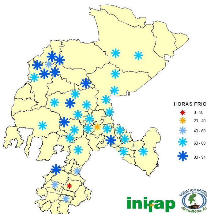
Figura 2. Horas frío acumuladas en la primera decena del mes de enero del 2018.
