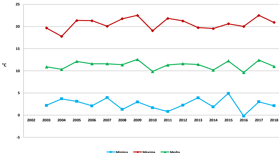
Figura 9. Temperatura promedio histórica en el mes de enero, considerando las 38 estaciones de la red de monitoreo agroclimático del estado de Zacatecas.
