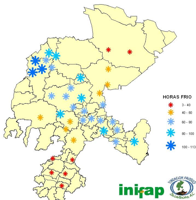
Figura 4. Horas frío acumuladas en la tercera decena del mes de enero del 2018.
