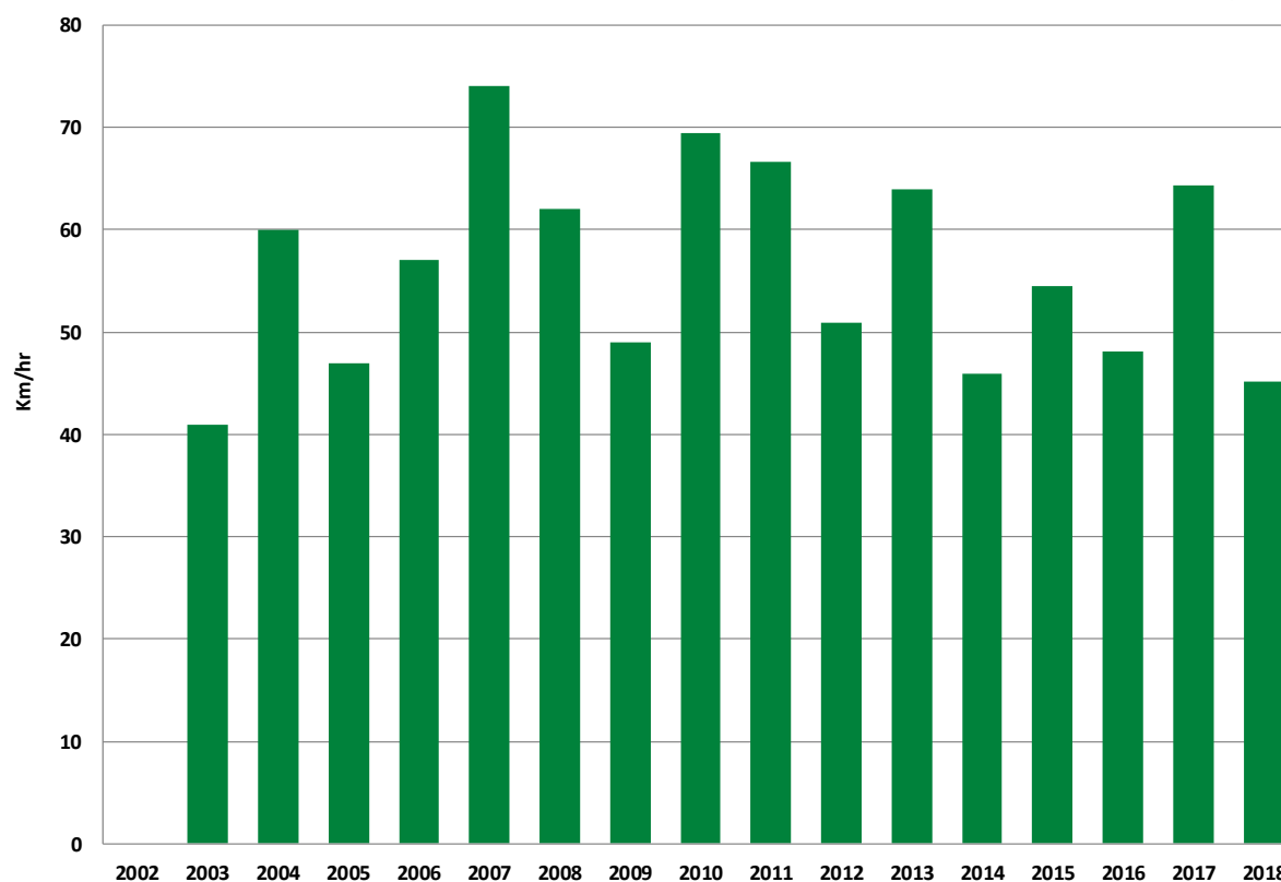
Figura 11. Valor máximo histórico de velocidad del viento en el mes de enero, considerando las 38 estaciones de la red de monitoreo agroclimático del estado de Zacatecas.
