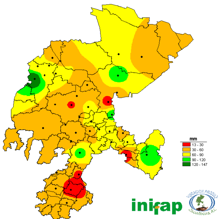
Figura 8. Precipitación de la segunda decena del mes de agosto del 2016. Red de monitoreo agroclimático del estado de Zacatecas.
