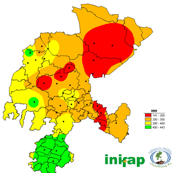
Figura 14. Precipitación acumulada en los meses de junio a agosto del 2016.
