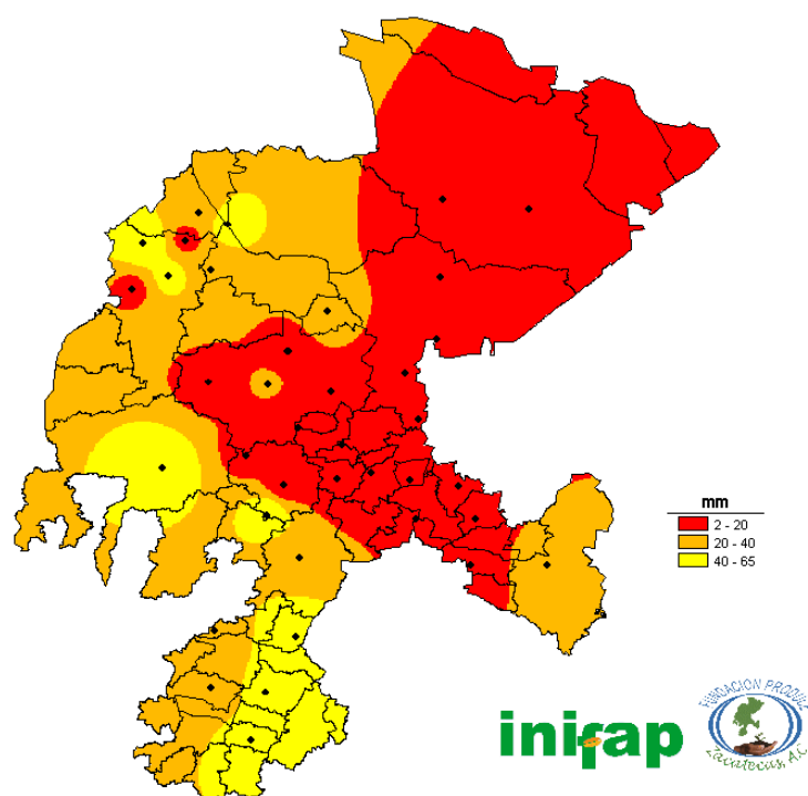
Figura 6. Precipitación de la primera decena del mes de agosto del 2016. Red de monitoreo agroclimático del estado de Zacatecas.
