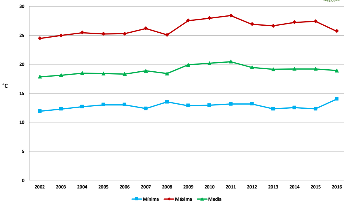
Figura 18. Temperaturas promedio histórica en el mes de agosto, considerando las 38 estaciones de la red de monitoreo agroclimático del estado de Zacatecas.
