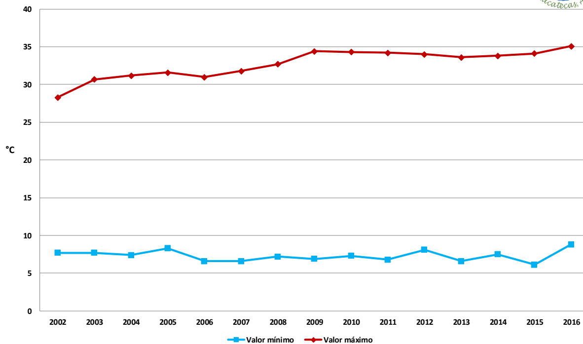
Figura 19. Valores máximos y mínimos históricos de temperatura en el mes de agosto, considerando las 38 estaciones de la red de monitoreo agroclimático del estado de Zacatecas.
