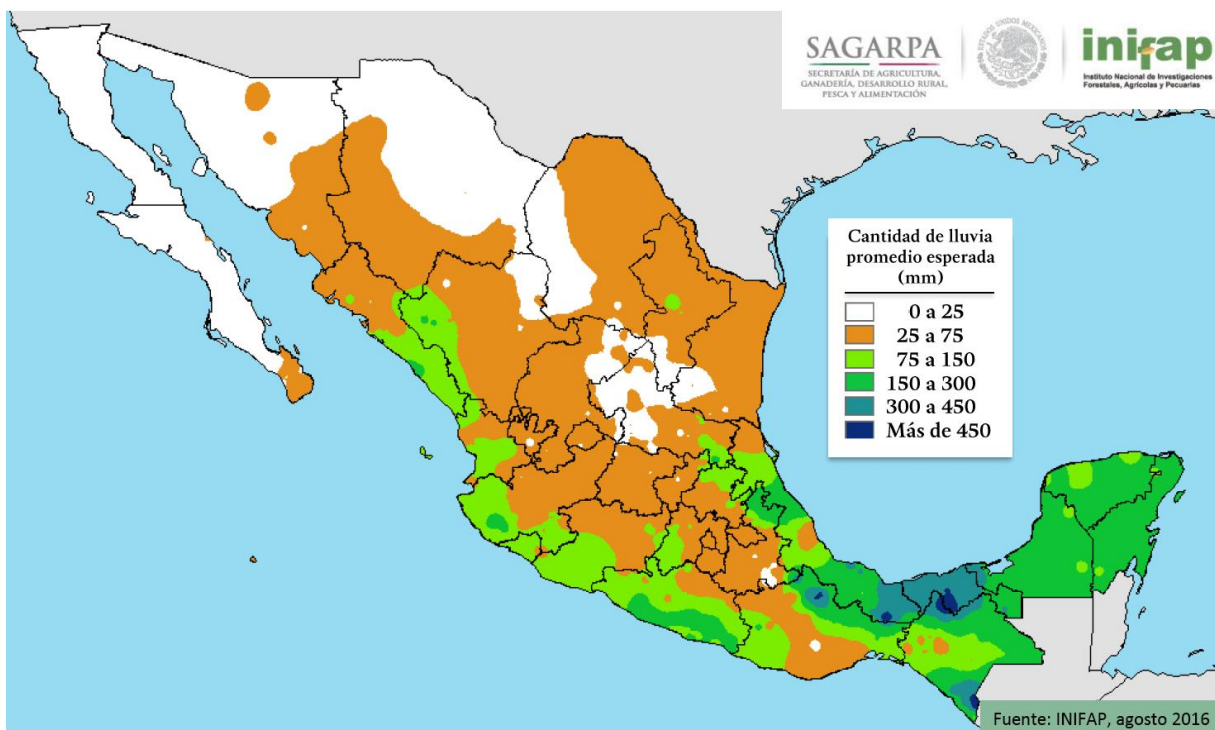
Figura 4. Pronóstico de lluvia para el mes de octubre de 2016.
