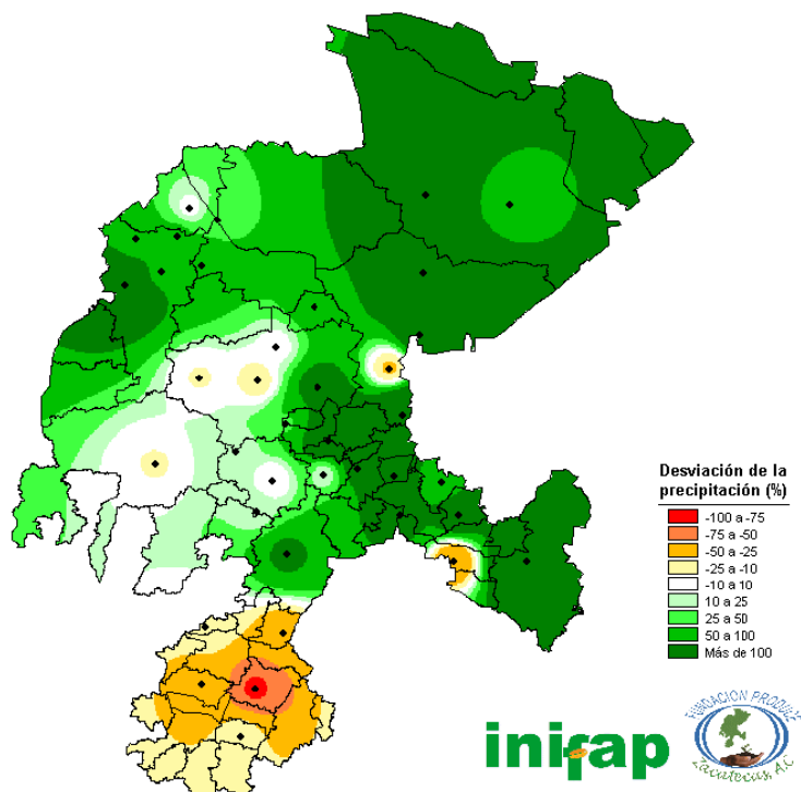
Figura 9. Porcentaje de la precipitación ocurrida en la segunda decena del mes de agosto del 2016 con respecto al promedio histórico. Red de monitoreo agroclimático del estado de Zacatecas.
