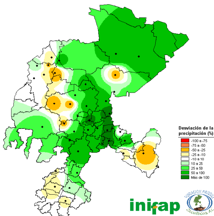
Figura 11. Porcentaje de la precipitación ocurrida en la tercera decena del mes de agosto del 2016 con respecto al promedio histórico. Red de monitoreo agroclimático del estado de Zacatecas.
