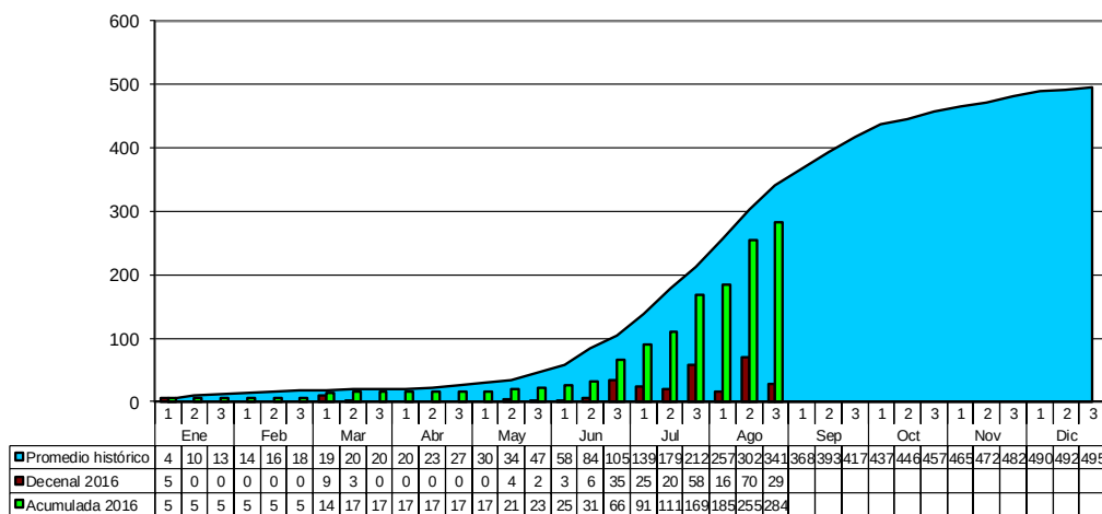
Figura 16. Precipitación decenal y acumulada hasta el mes de agosto en la estación Col. González Ortega, Sombrerete. Red de monitoreo agroclimático del estado de Zacatecas.
