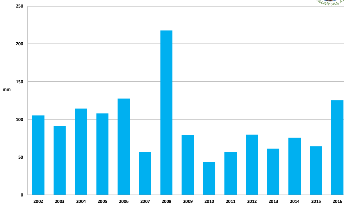
Figura 21. Precipitación promedio histórica del mes de agosto, considerando las 38 estaciones de la red de monitoreo agroclimático del estado de Zacatecas.
