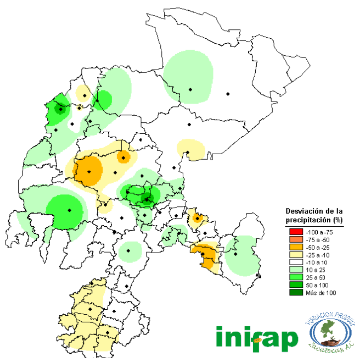
Figura 15. Porcentaje de la precipitación ocurrida en los meses de junio a agosto del 2016 con respecto al promedio histórico.
