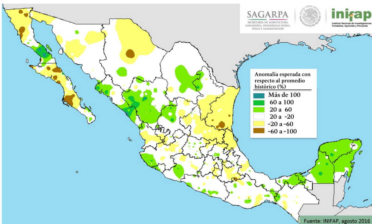
Figura 5. Pronóstico de anomalía de lluvia para el mes de octubre de 2016.
