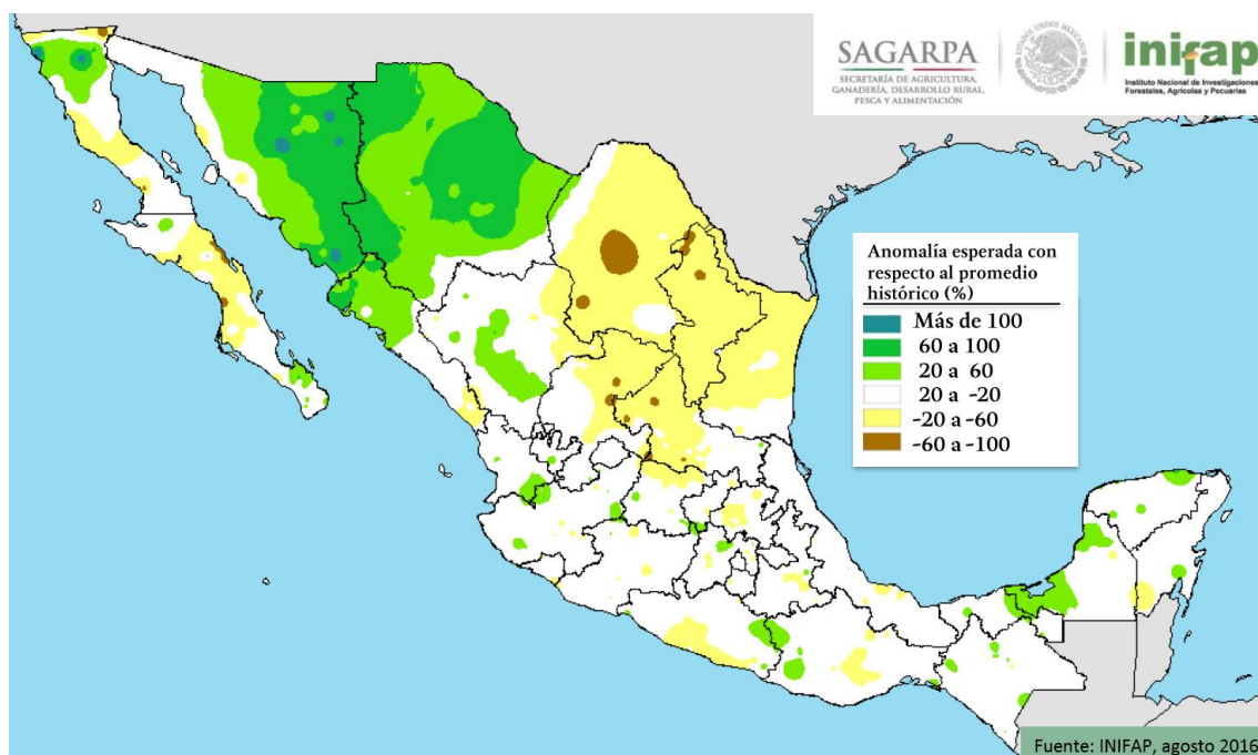
Figura 3. Pronóstico de anomalía de lluvia para el mes de septiembre de 2016.
