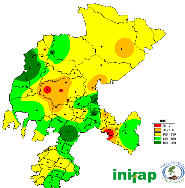
Figura 12. Precipitación del mes de agosto del 2016. Red de monitoreo agroclimático del estado de Zacatecas.
