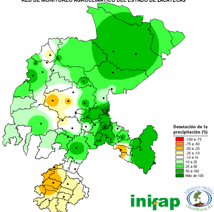
Figura 13. Porcentaje de la precipitación ocurrida en el mes de agosto del 2016 con respecto al promedio histórico. Red de monitoreo agroclimático del estado de Zacatecas.
