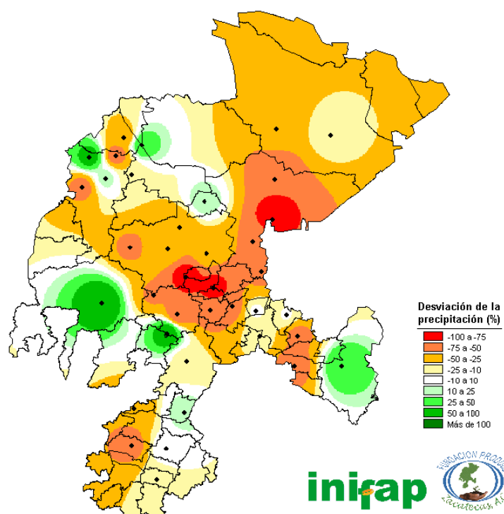
Figura 7. Porcentaje de la precipitación ocurrida en la primera decena del mes de agosto del 2016 con respecto al promedio histórico. Red de monitoreo agroclimático del estado de Zacatecas.
