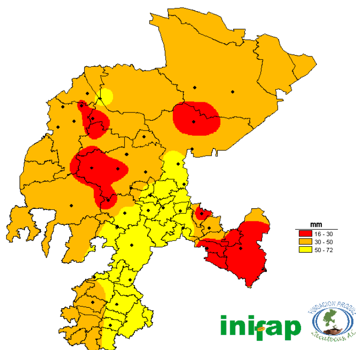
Figura 10. Precipitación de la tercera decena del mes de agosto del 2016. Red de monitoreo agroclimático del estado de Zacatecas.
