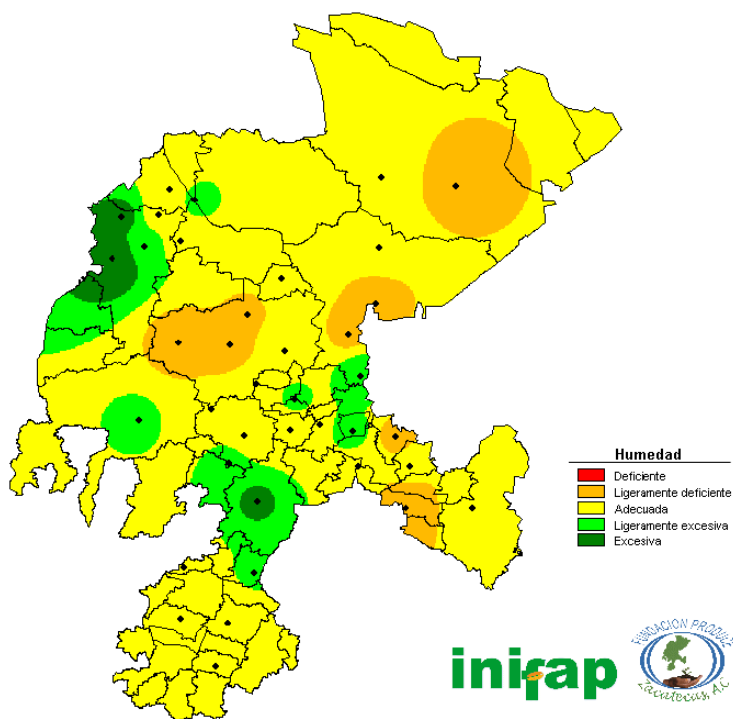
Figura 17. Índice de humedad del mes de agosto del 2016.
