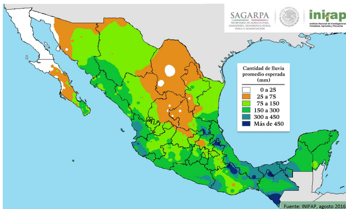
Figura 2. Pronóstico de lluvia para el mes de septiembre de 2016.
