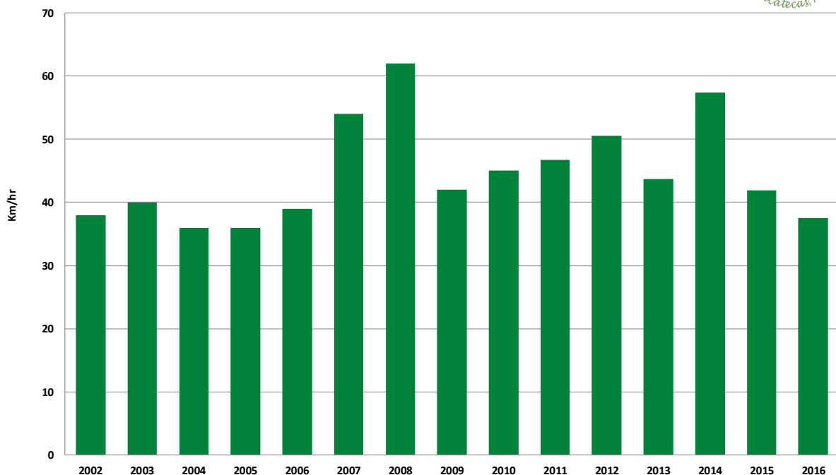
Figura 20. Valor máximo histórico de velocidad del viento en el mes de agosto, considerando las 38 estaciones de la red de monitoreo agroclimático del estado de Zacatecas.
