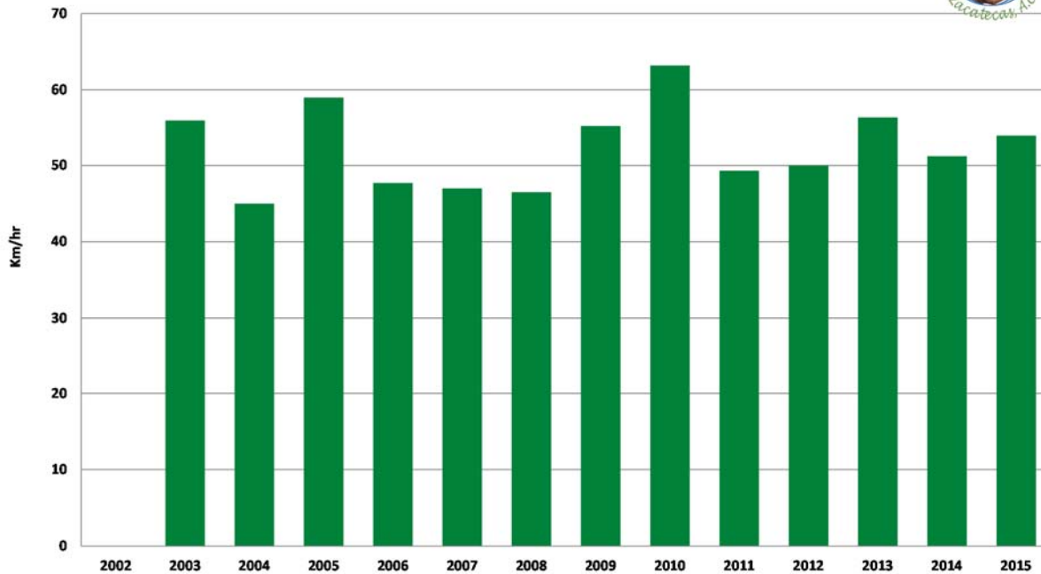
FIGURA 10. VALOR MÁXIMO DE VELOCIDAD DEL VIENTO EN EL MES DE ABRIL, CONSIDERANDO LAS 36 ESTACIONES DE LA RED DE MONITOREO AGROCLIMÁTICO DEL ESTADO DE ZACATECAS.
