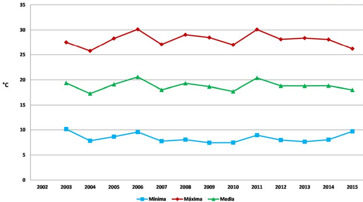
FIGURA 9. TEMPERATURAS PROMEDIO EN EL MES DE ABRIL, CONSIDERANDO LAS 36 ESTACIONES DE LA RED DE MONITOREO AGROCLIMÁTICO DEL ESTADO DE ZACATECAS.
