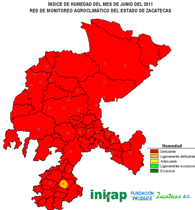
FIGURA 11. Índice de humedad del mes de junio del 2011.
