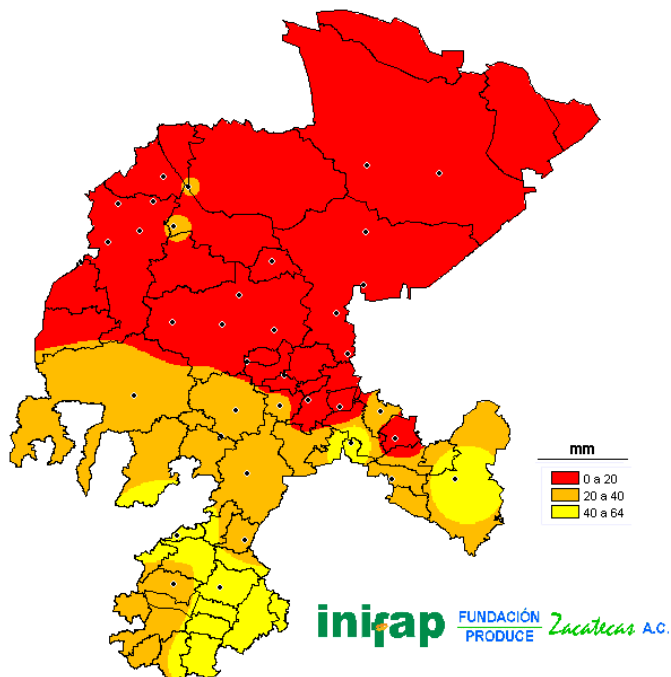
FIGURA 6. Precipitación de la tercera decena de junio del 2011.
