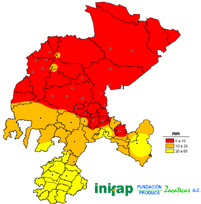
FIGURA 8. Precipitación del mes de junio del 2011.
