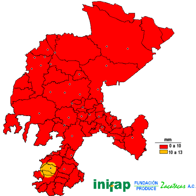
FIGURA 2. Precipitación de la primera decena de junio del 2011.
