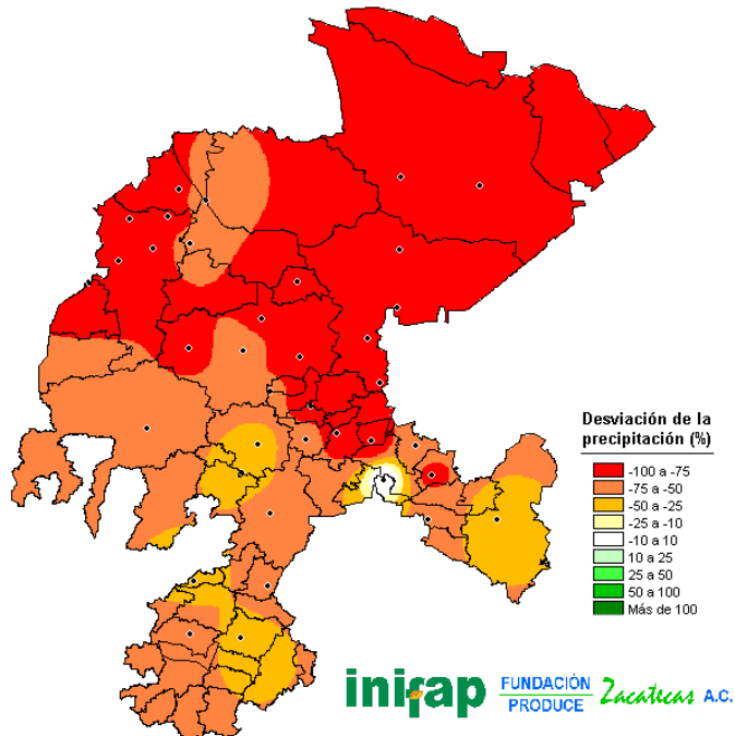
FIGURA 9. Porcentaje de la precipitación ocurrida en el mes de junio del 2011 con respecto al promedio histórico.
