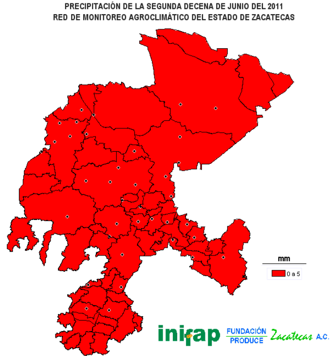
FIGURA 4. Precipitación de la segunda decena de junio del 2011.
