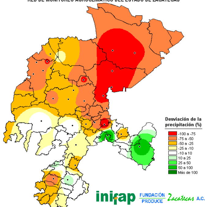
FIGURA 7. Porcentaje de la precipitación ocurrida en la tercera decena del mes de junio del 2011 con respecto al promedio histórico.
