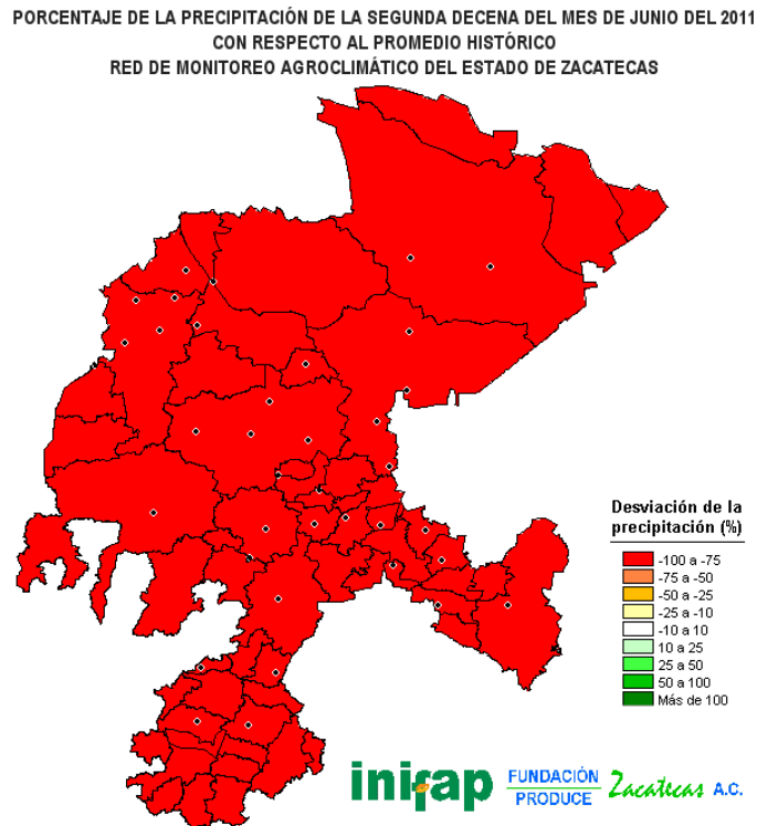
FIGURA 5. Porcentaje de la precipitación ocurrida en la segunda decena del mes de junio del 2011 con respecto al promedio histórico.
