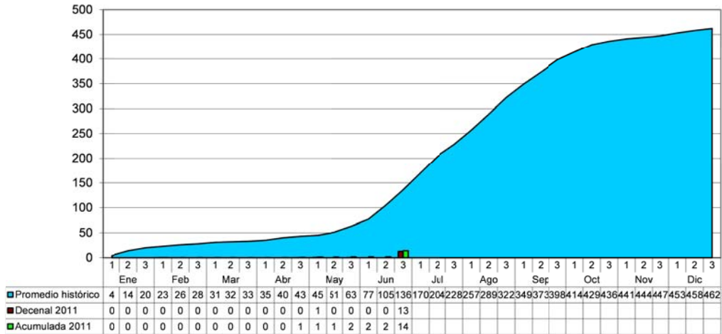
FIGURA 10. Precipitación decenal y acumulada hasta el mes de junio en la estación U. A. Biología, Guadalupe.
