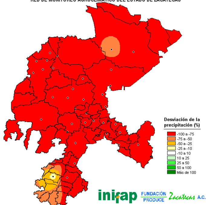
FIGURA 3. Porcentaje de la precipitación ocurrida en la primera decena del mes de junio del 2011 con respecto al promedio histórico.
