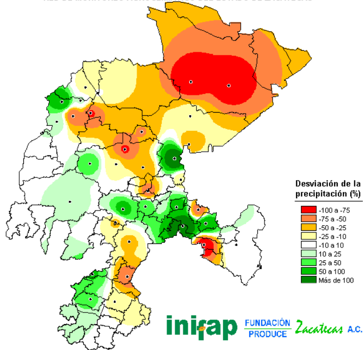
FIGURA 7. Porcentaje de la precipitación ocurrida en la tercera decena del mes de julio del 2010 con respecto al promedio histórico.
