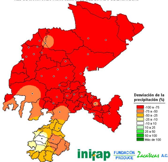
FIGURA 5. Porcentaje de la precipitación ocurrida en la segunda decena del mes de julio del 2010 con respecto al promedio histórico.
