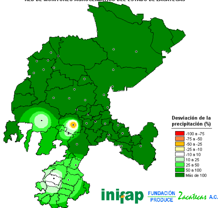
FIGURA 3. Porcentaje de la precipitación ocurrida en la primera decena del mes de julio del 2010 con respecto al promedio histórico.
