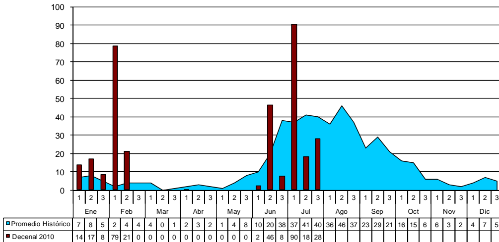
FIGURA 10. Precipitación decenal y acumulada hasta el mes de julio en la estación Villanueva, Villanueva.
