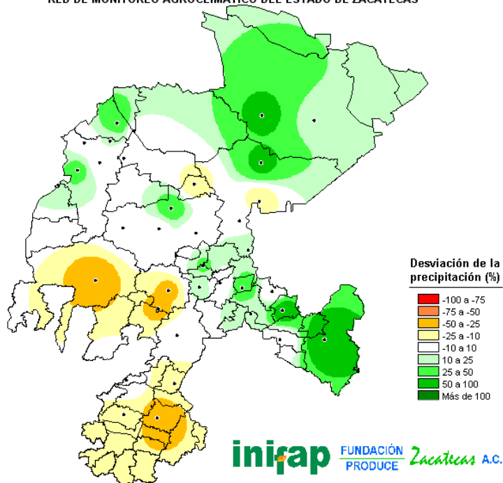
FIGURA 11. Porcentaje de la precipitación ocurrida en los meses de junio a julio del 2010 con respecto al promedio histórico.
