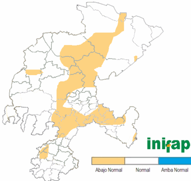
FIGURA 12. Pronóstico de lluvia para el mes de julio del 2010.
