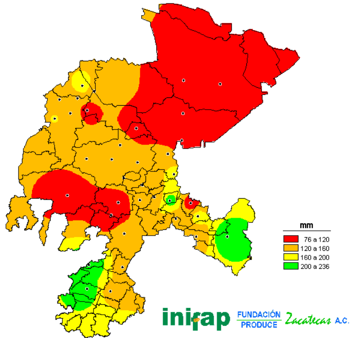
FIGURA 8. Precipitación del mes de julio del 2010.
