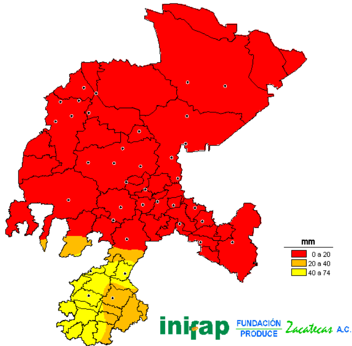
FIGURA 4. Precipitación de la segunda decena de julio del 2010.
