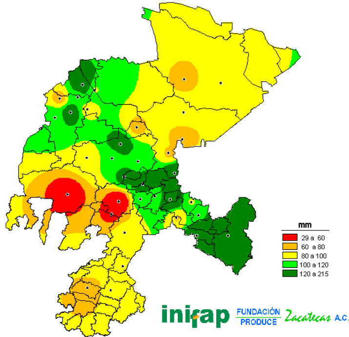
FIGURA 2. Precipitación de la primera decena de julio del 2010.
