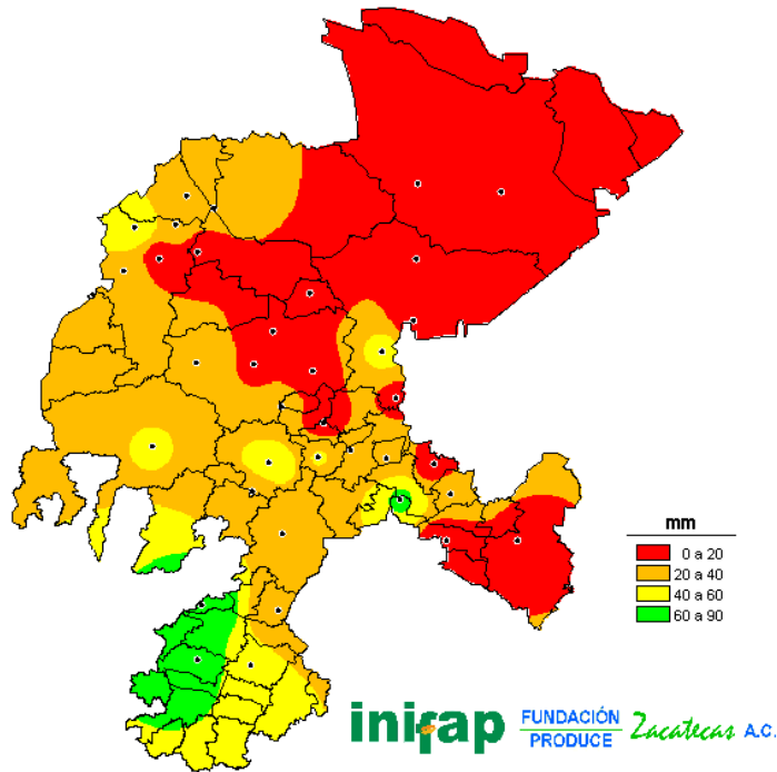
FIGURA 6. Precipitación de la tercera decena de julio del 2010.
