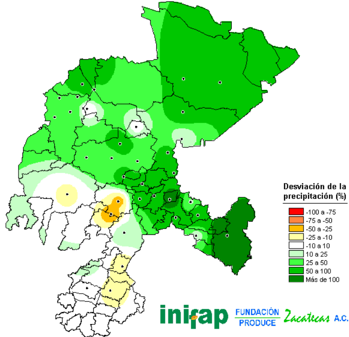
FIGURA 9. Porcentaje de la precipitación ocurrida en el mes de julio del 2010 con respecto al promedio histórico.
