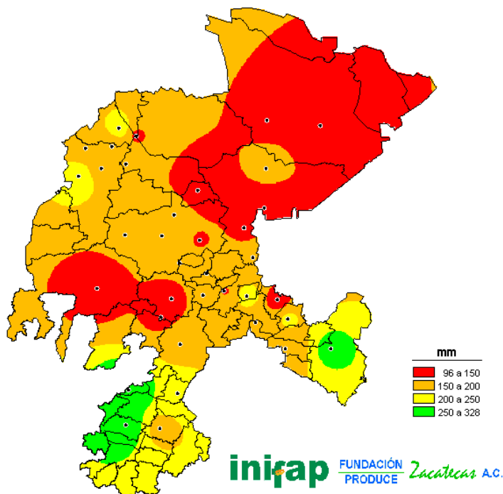
FIGURA 10. Precipitación acumulada en los meses de junio a julio del 2010.
