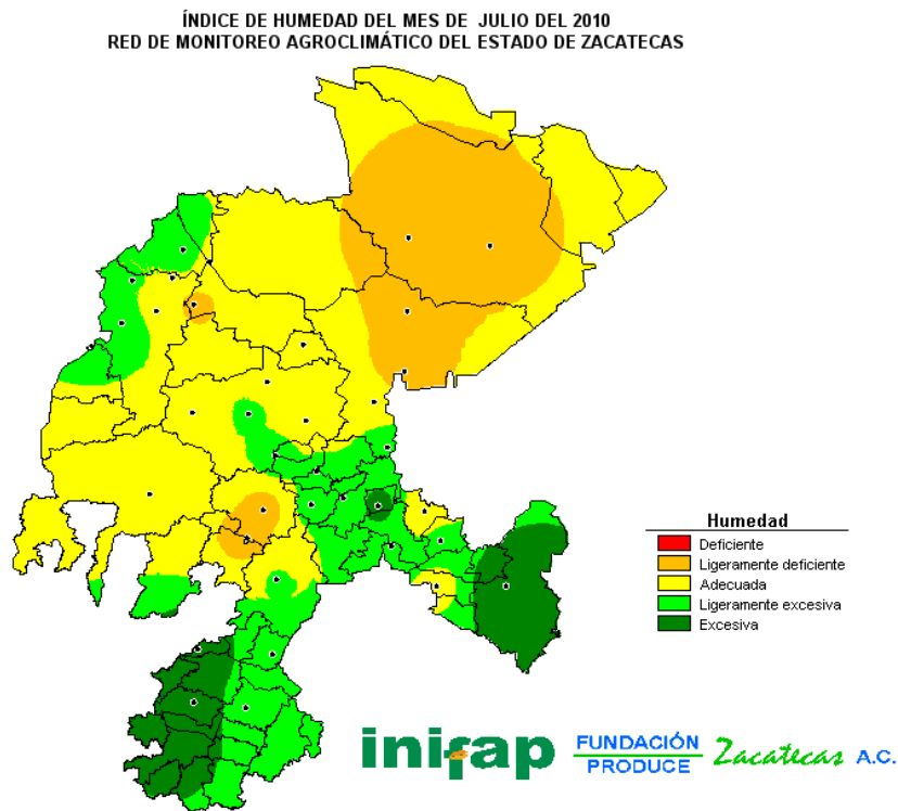
FIGURA 14. Índice de humedad del mes de julio del 2010.
