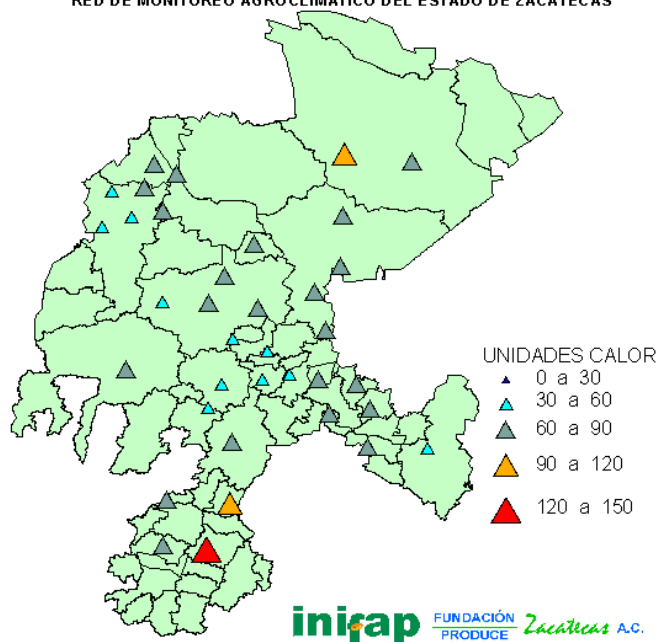
FIGURA 4. Unidades calor de la tercera decena del mes de marzo del 2009.
