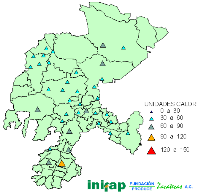
FIGURA 2. Unidades calor de la primera decena del mes de marzo del 2009.
