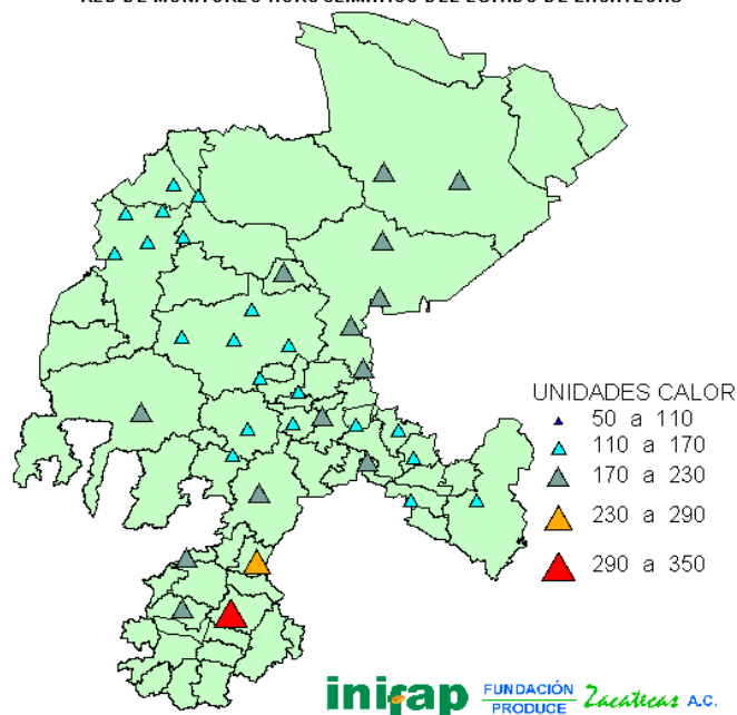
FIGURA 5. Unidades calor acumuladas durante el mes de marzo del 2009.
