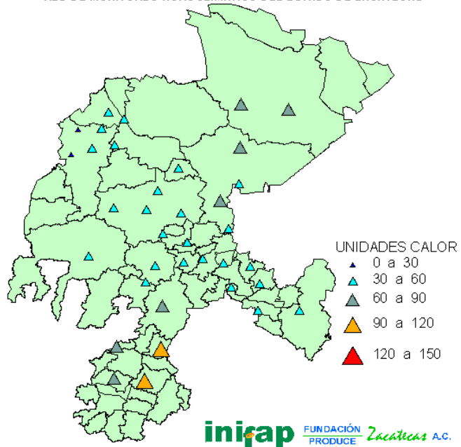
FIGURA 3. Unidades calor de la segunda decena del mes de marzo del 2009.
