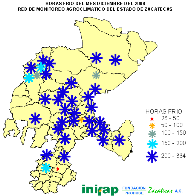
FIGURA 5. Horas frío acumuladas en el mes de diciembre del 2008.
