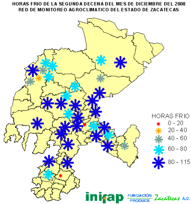
FIGURA 3. Horas frío acumuladas en la segunda decena del mes de diciembre del 2008.
