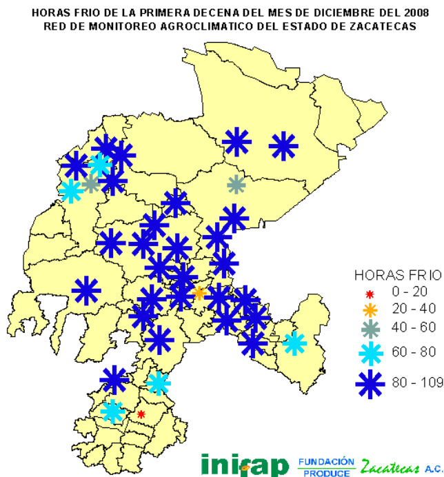
FIGURA 2. Horas frío acumuladas en la primera decena del mes de diciembre del 2008.
