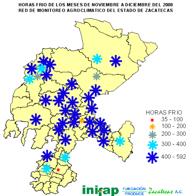
FIGURA 6. Horas frío acumuladas durante los meses de noviembre a diciembre del 2008.
