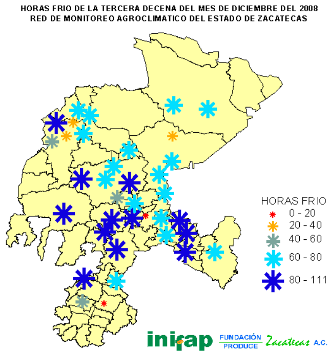
FIGURA 4. Horas frío acumuladas en la tercera decena del mes de diciembre del 2008.
