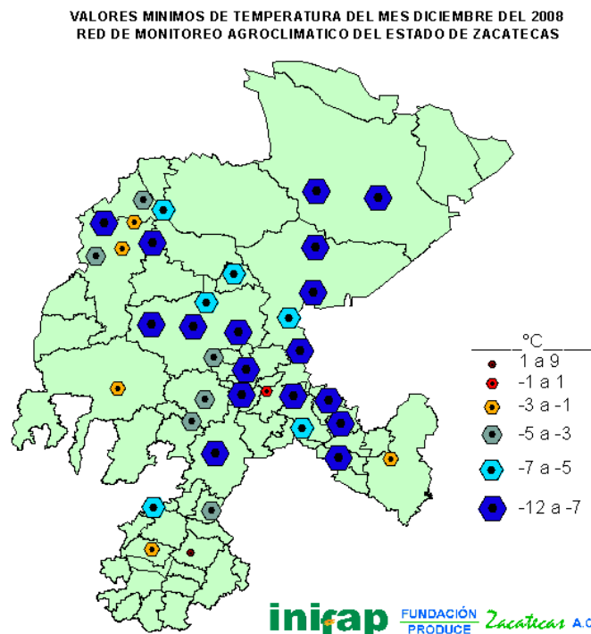
FIGURA 8. Valores mínimos de temperatura registrados en el mes de diciembre del 2008.
