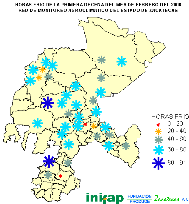
FIGURA 2. Horas frío acumuladas en la primera decena del mes de febrero del 2008.
