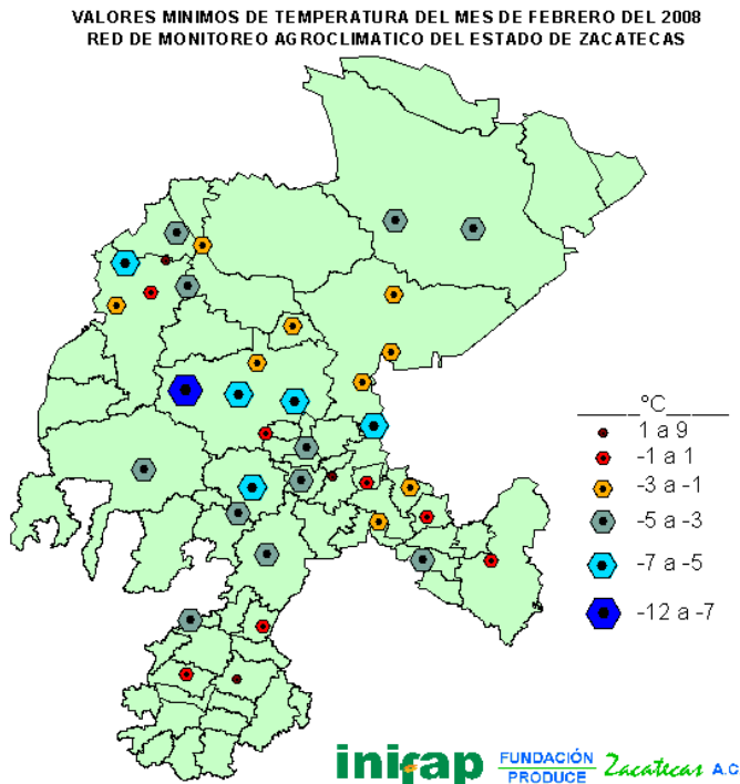
FIGURA 8. Valores mínimos de temperatura registrados en el mes de febrero del 2008.
