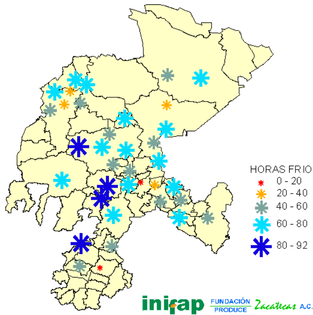
FIGURA 3. Horas frío acumuladas en la segunda decena del mes de febrero del 2008.
