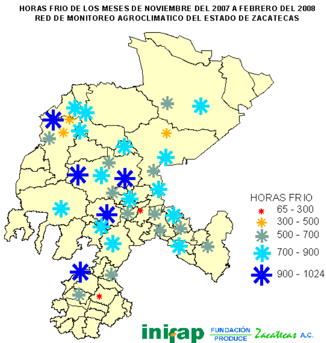
FIGURA 6. Horas frío acumuladas durante los meses de noviembre a febrero del 2008
