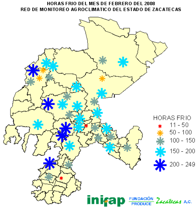
FIGURA 5. Horas frío acumuladas en el mes de febrero del 2008.
