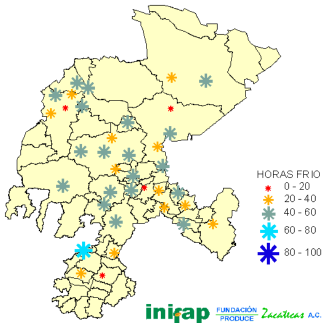
FIGURA 4. Horas frío acumuladas en la tercera decena del mes de febrero del 2008.
