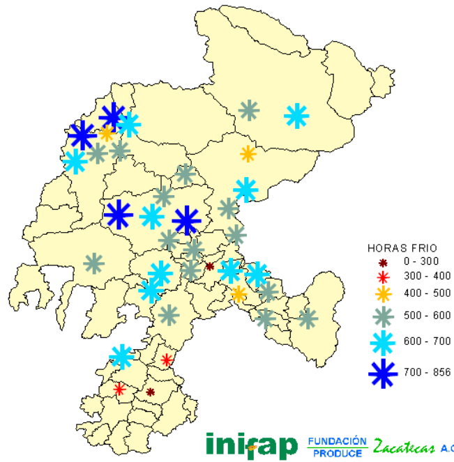
FIGURA 6. Horas frío acumuladas en los meses de noviembre del 2006 a enero del 2007.
