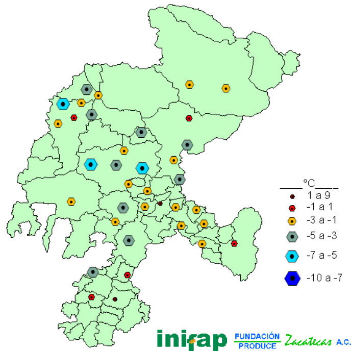
FIGURA 7. Valores mínimos de temperatura registrados en el mes de enero del 2007.
