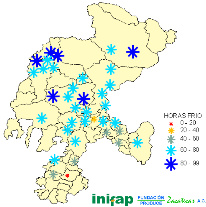
FIGURA 2. Horas frío acumuladas en la primera decena del mes de enero del 2007.
