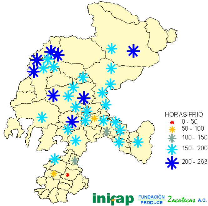
FIGURA 5. Horas frío acumuladas en el mes de enero del 2007.
