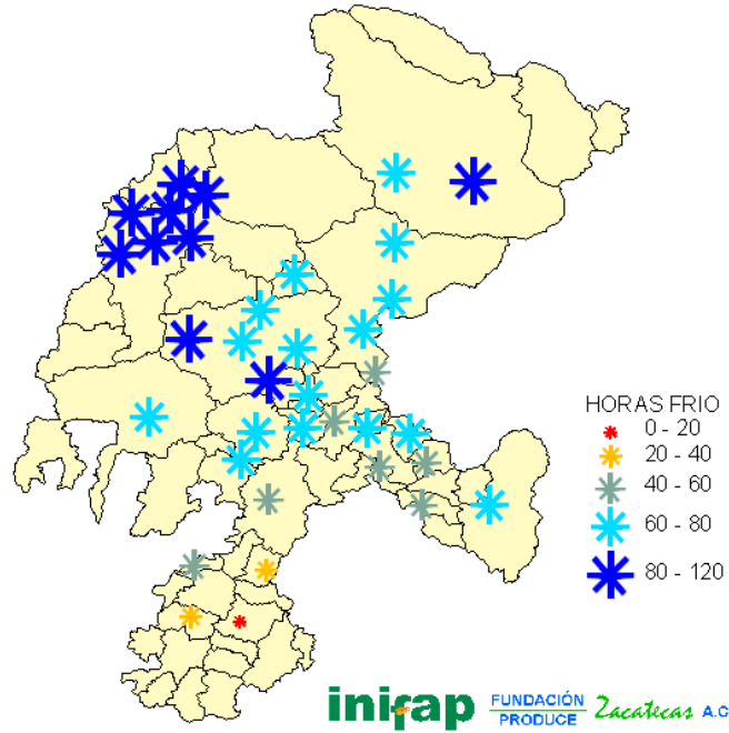
FIGURA 4. Horas frío acumuladas en la tercera decena del mes de enero del 2007.
