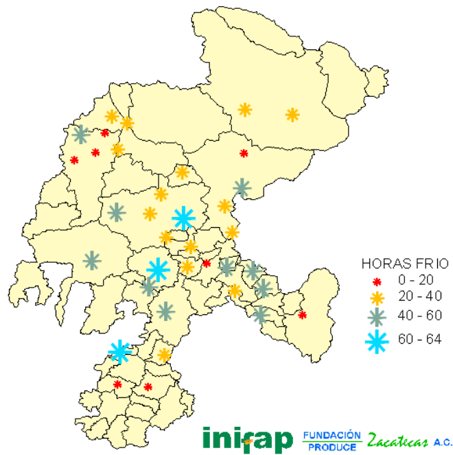
FIGURA 3. Horas frío acumuladas en la segunda decena del mes de enero del 2007.
